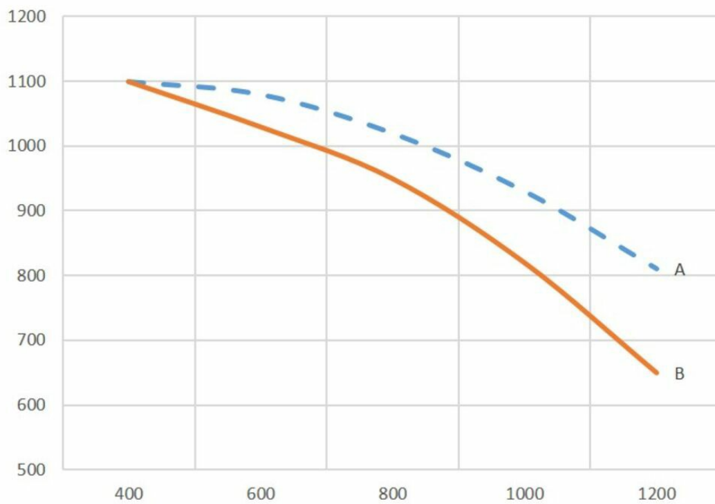
A: Wentylator - całkowite ciśnienie B: Wentylator - ciśnienie statyczne X: m 3 /h Y: Pa
