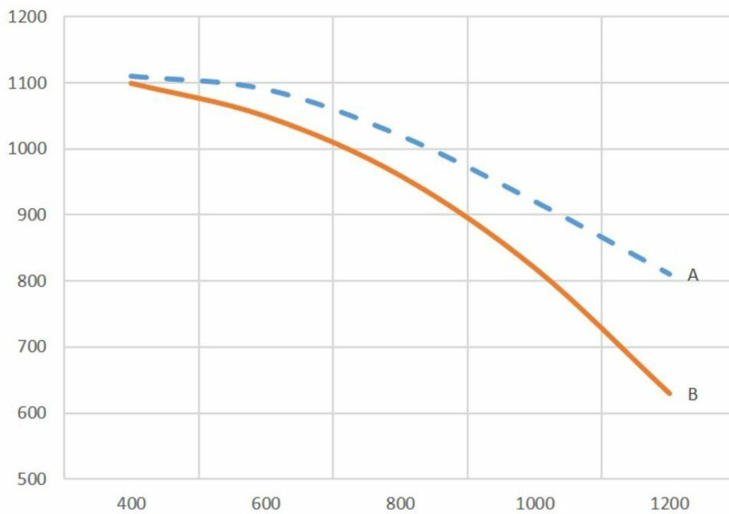
A: Ciężnienie całkowite wentylatora B: Ciężnienie statyczne wentylatora X: m 3 /h Y: Pa
