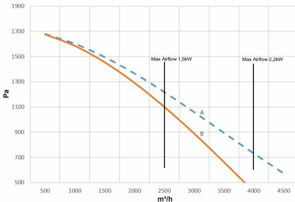
A: Ciśnienie całkowite B: Ciśnienie statyczne X: m³/h Y: Pa
